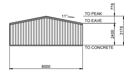
3 7 ENDWALL EXTERIOR ELEVATION SCALE: 1 = 250
